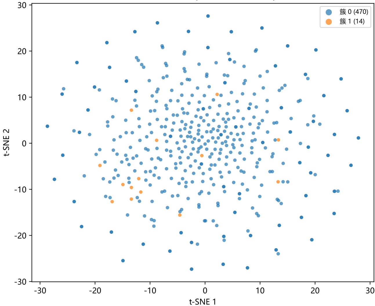
t-SNE 聚类着色 (K-Means++ K=2)
