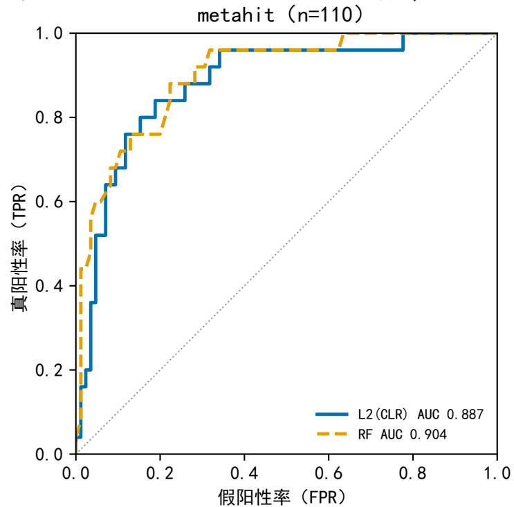
三数据集 ROC 曲线 (L2+CLR 主模型与 RF 对照, 5 折 CV 00F)
