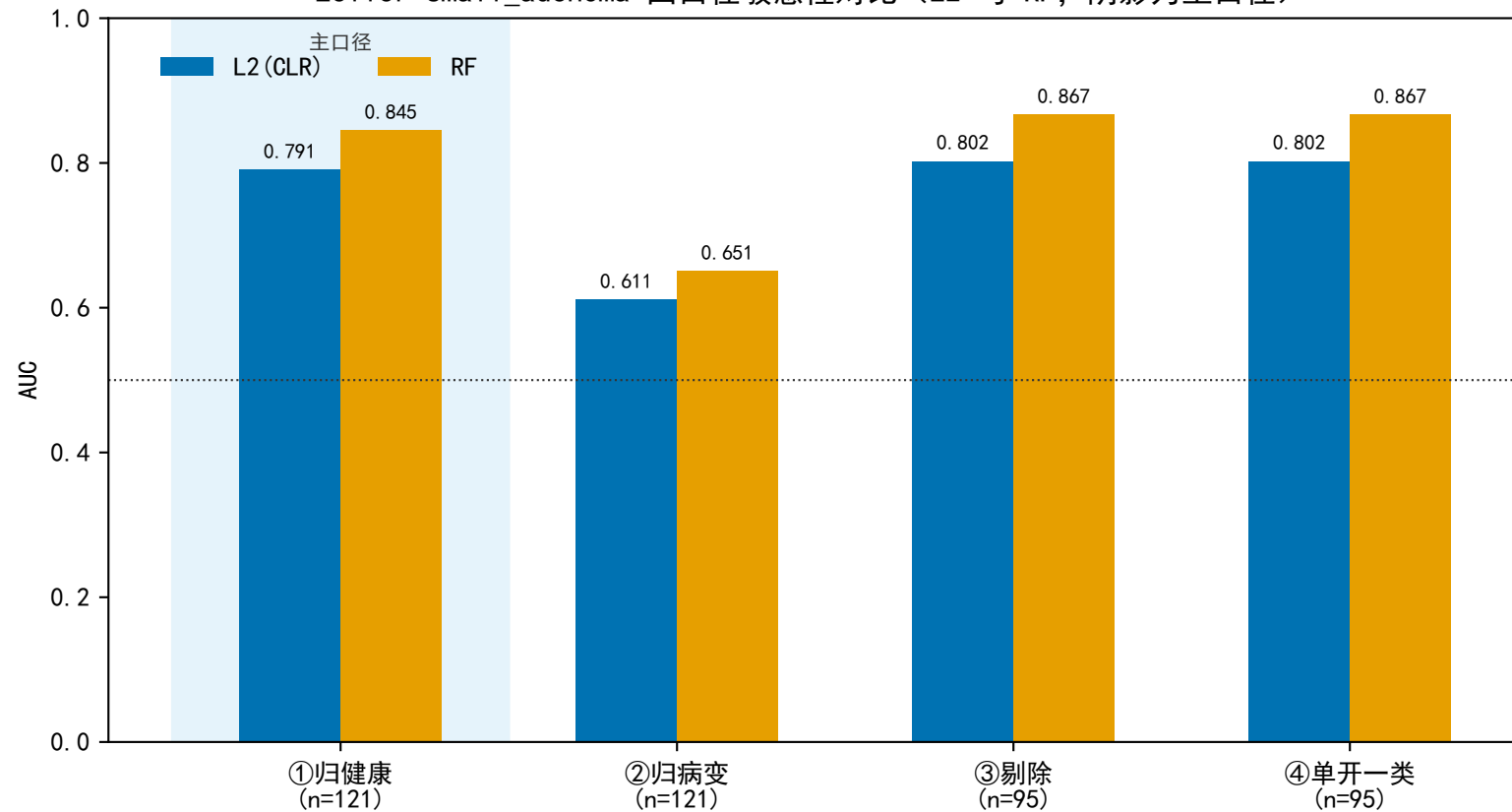
Zeller_small_adenoma 四口径敏感性对比 (L2 与 RF, 阴影为主口径)
