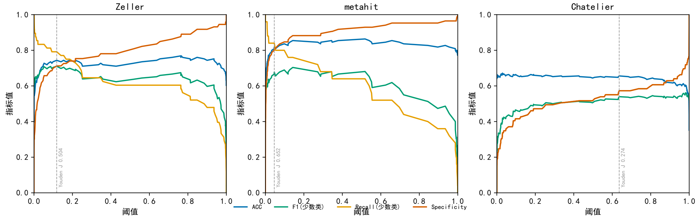
L2 主模型阈值-指标曲线 (5 折 CV 00F, 虚线为 Youden 最优阈值)
