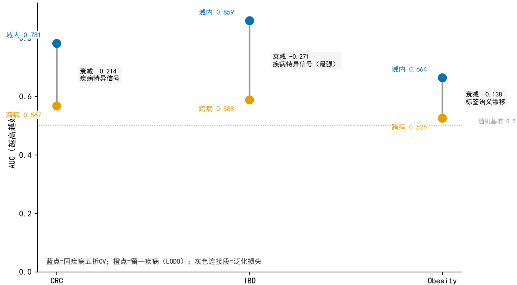
跨疾病泛化造成的 AUC 下降：域内性能与 LODO 性能对照
