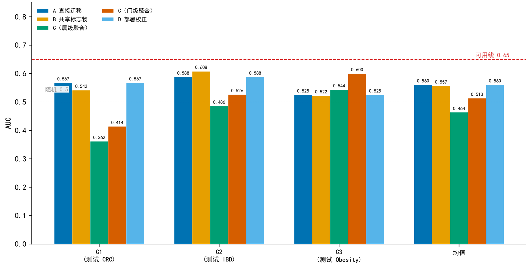
五种策略配置在 3 个 LOD0 组合及其均值下的 AUC 对比
