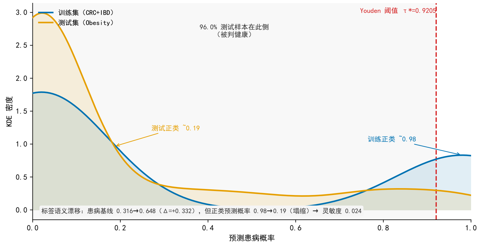
C3 阈值漂移：测试概率分布左移导致阈值失准
