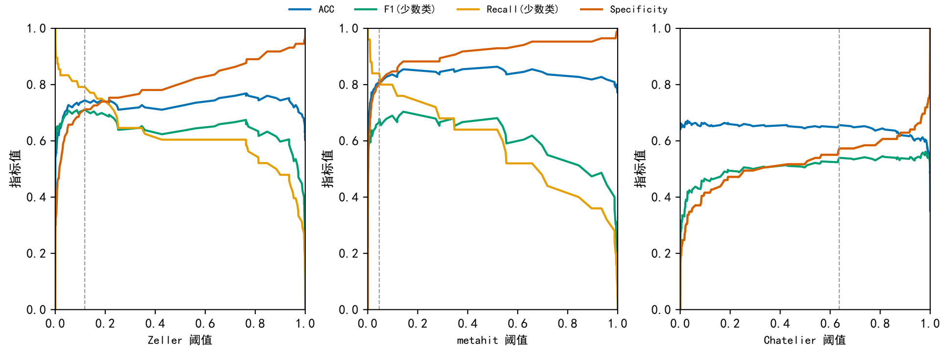
L2 主模型阈值-指标曲线 (5 折 CV 00F, 虚线为 Youden 最优阈值)
