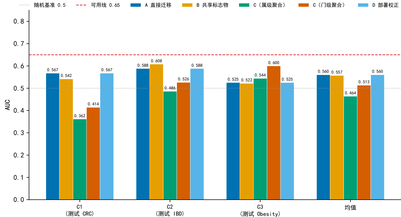
五种策略配置在 3 个 LOD0 组合及其均值下的 AUC 对比
