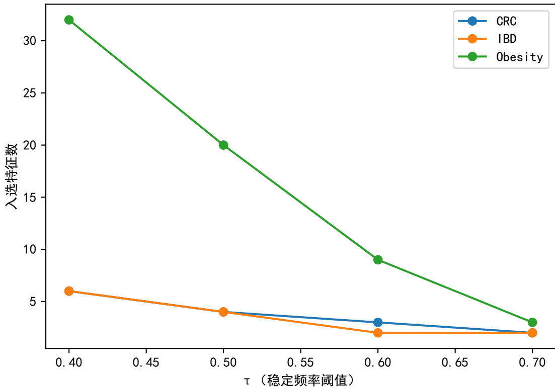
\tau 敏感性：入选特征数随 \tau 变化
