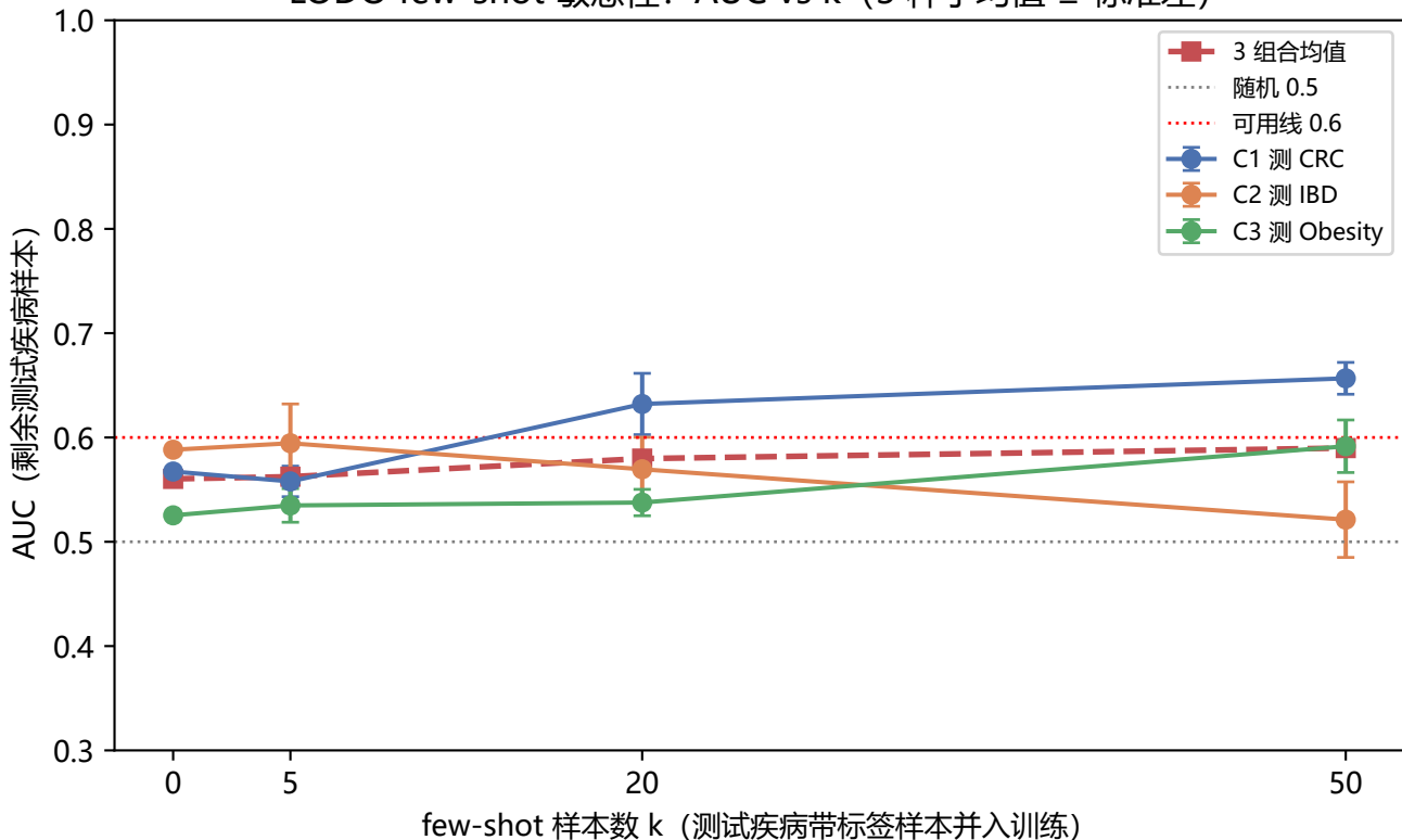
LODO few-shot 敏感性: AUC vs k (3 种子均值 \pm 标准差)
