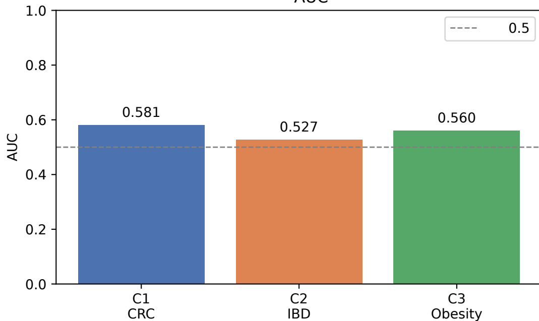
AUC
