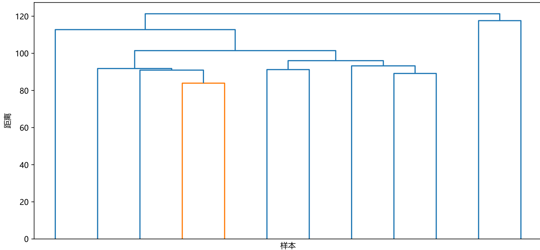
层次聚类树状图 (Ward 法, PCA 空间)
