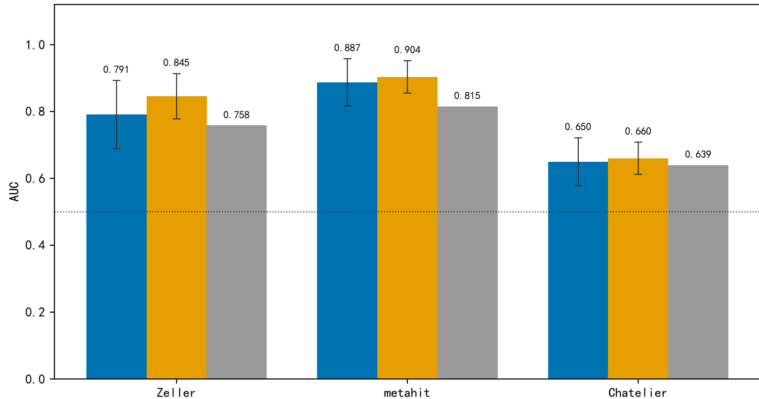
三数据集 L2 / RF / 单特征基线 AUC 对比 (5 折 CV, 误差棒表示折间标准差)
