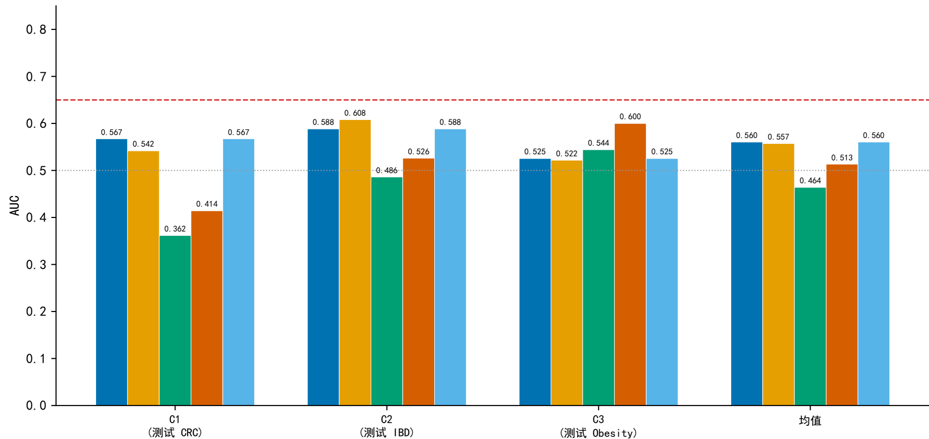
五种策略配置在 3 个 LODO 组合及其均值下的 AUC 对比
