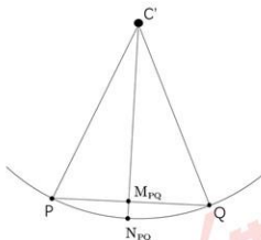
图七: 球心、圆弧中点坐标的求解
