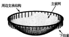
图 1 FAST 主动反射面轴侧图
