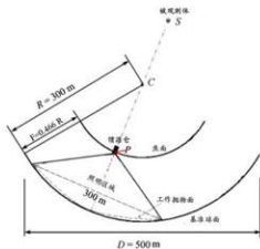
图 6 FAST 剖面示意图
