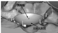
图 2 FAST 三维位置示意图
