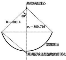
图 16 照明区域基准球面的几何关系
