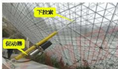
图 3 下拉索和促动器实物图
