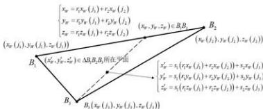
图 9: 反馈面板三角形区域示意图
