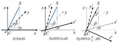
图 6: 坐标系旋转示意图
