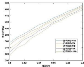
图20. 终止时刻随螺旋的螺距和把手间距的变化曲线图
