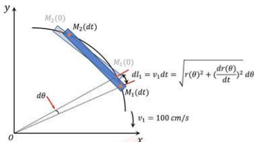
图3 螺旋线弧长的积分求解
