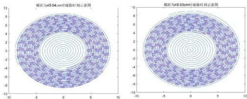
图 22 螺距为 45.04cm 时碰撞时刻示意图
