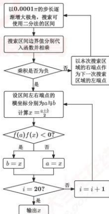
图7 二分法求解龙头前把手位置流程图
