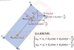
图 13 板凳顶点的推导
