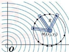
图4 圆和螺旋线方程的联立
