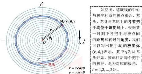
图2 极坐标系中的阿基米德螺旋线
