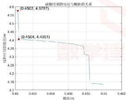
图 21 小步长遍历搜索螺距
