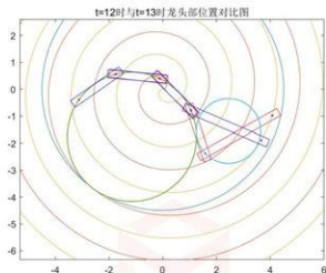
图 27 第 12 s~13 s 龙头部分的轨迹图
