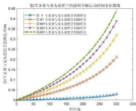
图 9 把手路程差随时间变化的图像
