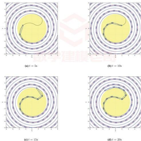
图 20 调头过程中不同时刻板凳龙示意图
