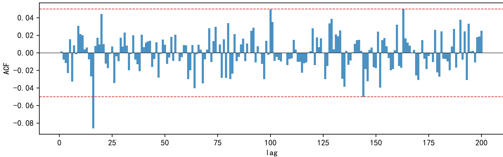
ACF (Total, lag1-200) \approx 0 \rightarrow 白噪声
