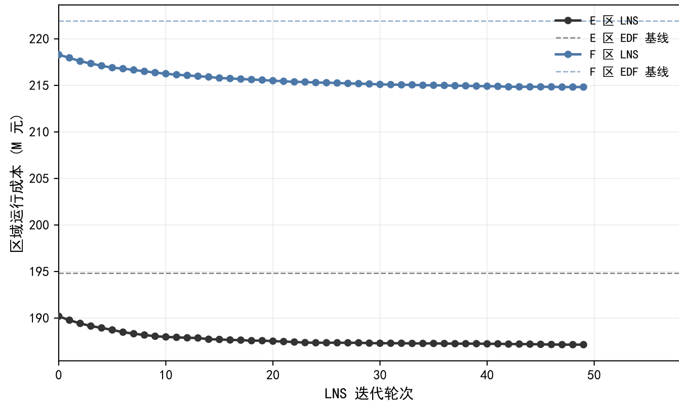
LNS 大邻域搜索收敛曲线 (E/F 区, 50 轮)
