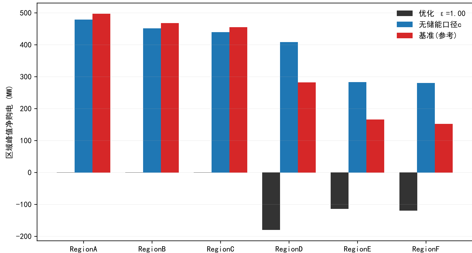
区域峰值净购电削峰效果（主时域）
