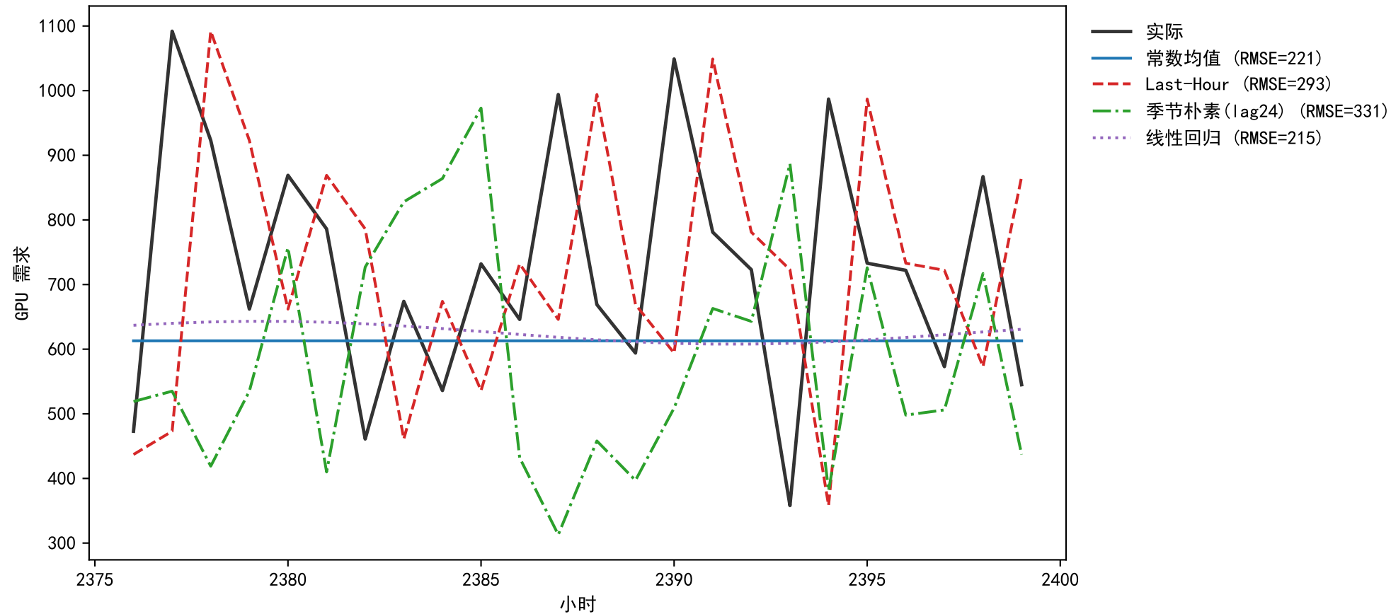
测试窗 2376-2399 预测 vs 实际 (4 基线)
