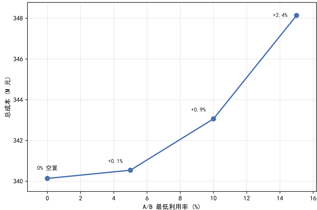
区域最低利用率 vs 总成本 (A/B 保底承接灵敏度)
