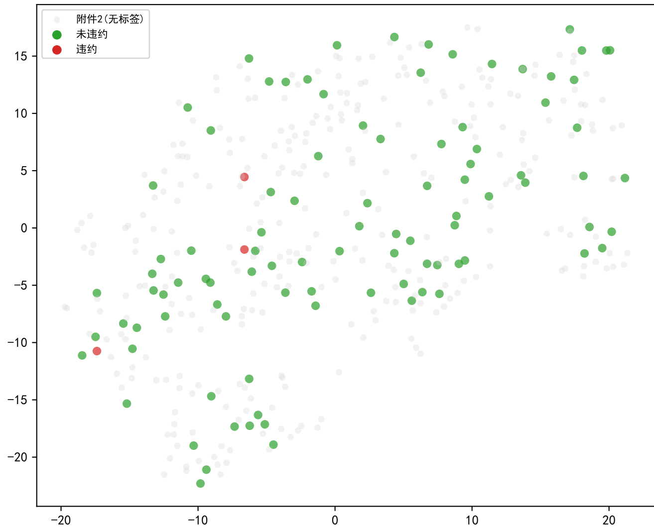
违约标签对照 (t-SNE)
