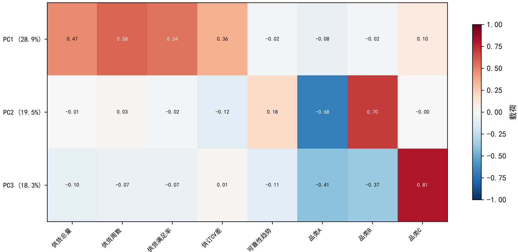
PCA 主成分载荷 v2
