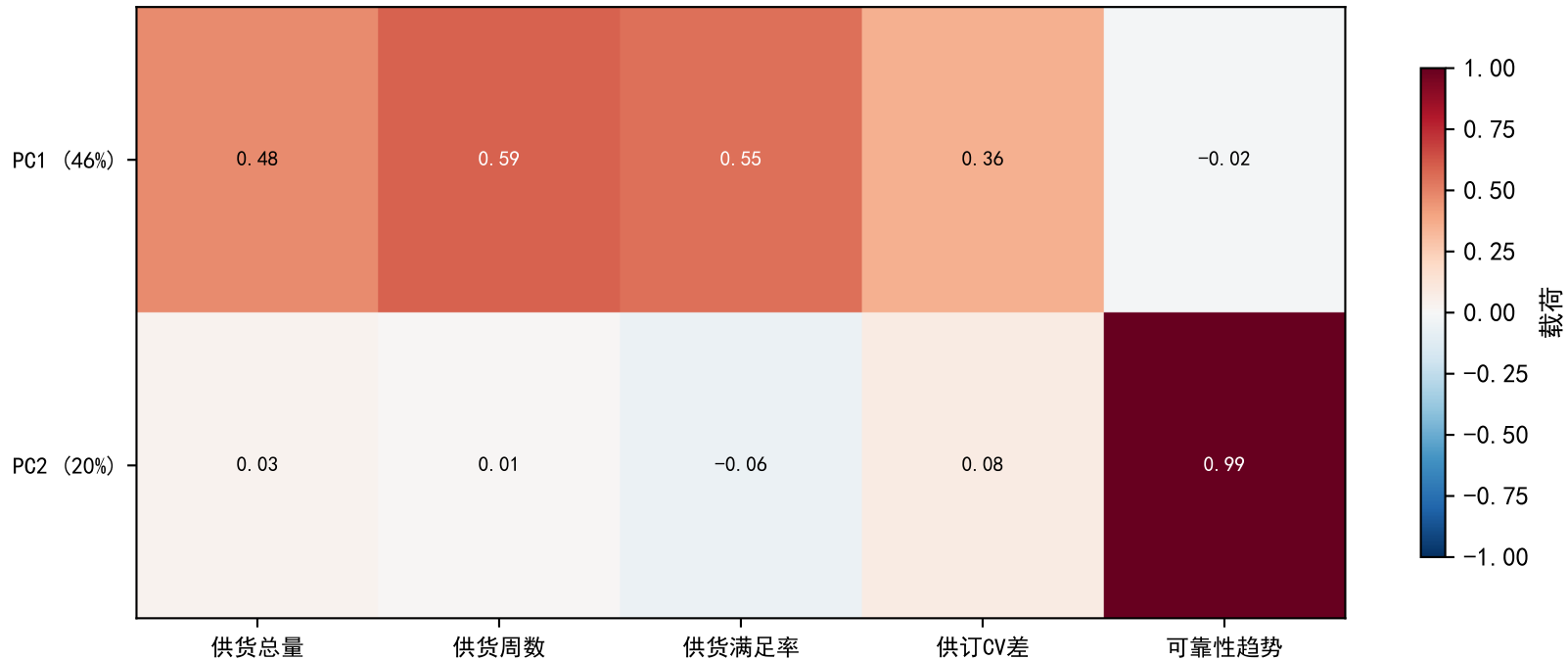
PCA 主成分载荷矩阵
