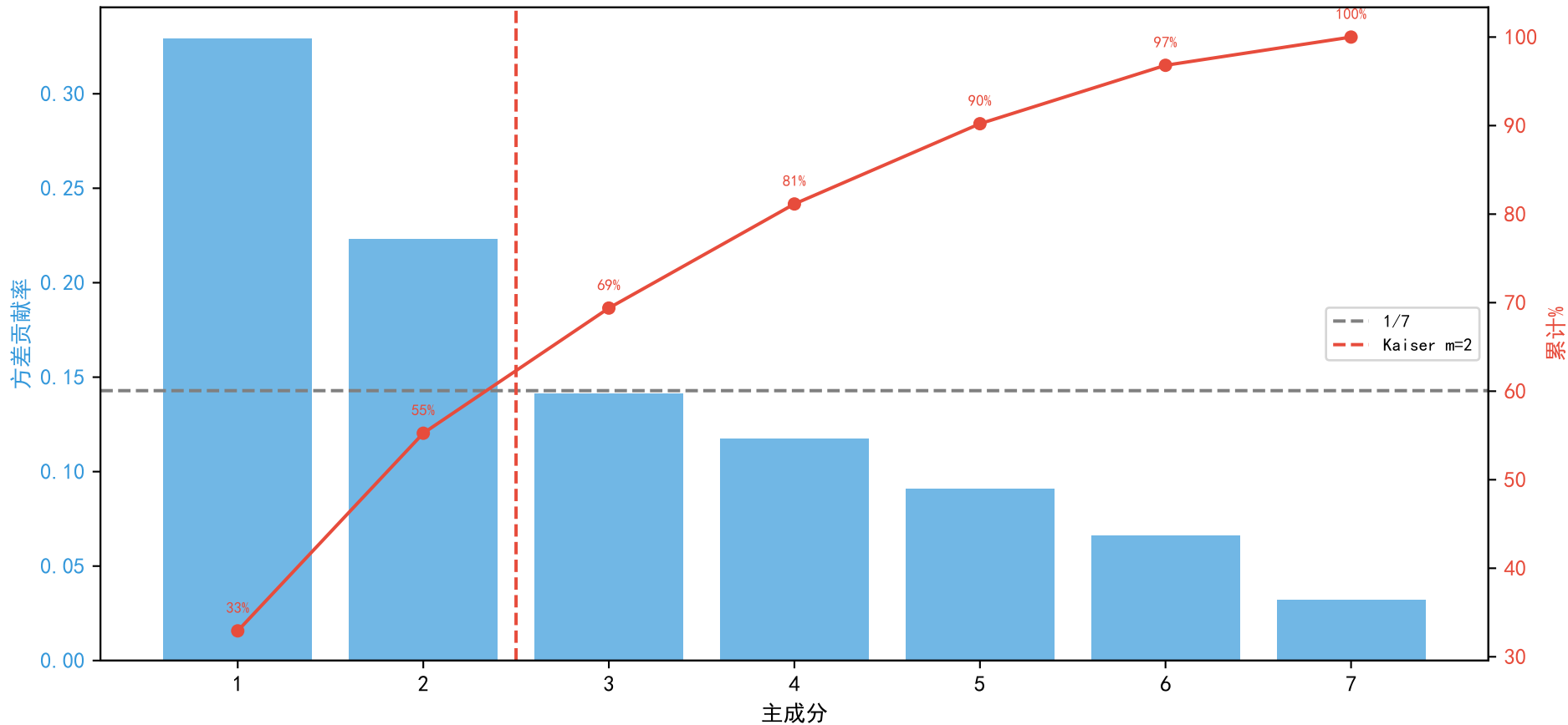
PCA 碎石图 v3 (m=2, 累计55.3%)
