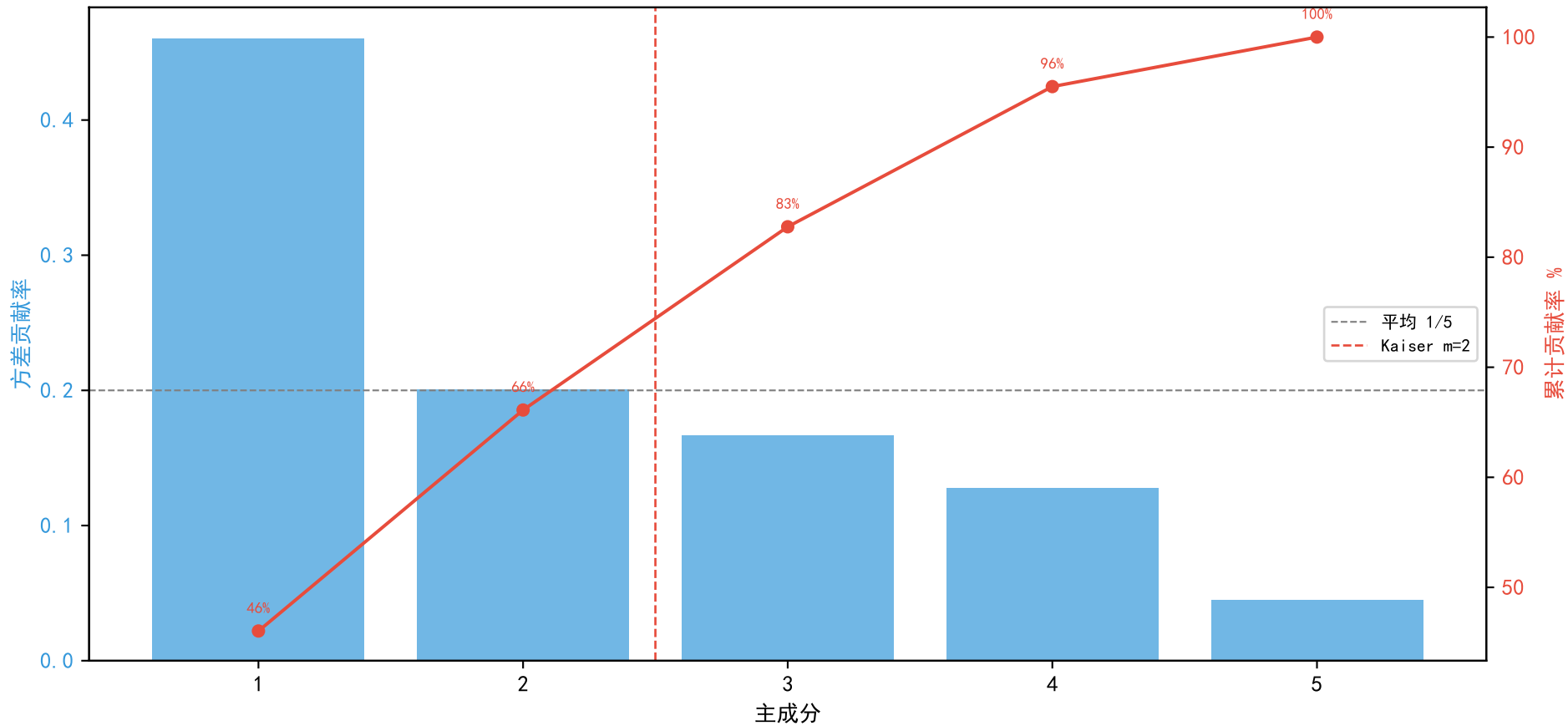
PCA 碎石图 (Kaiser m=2, 累计 66.1%)
