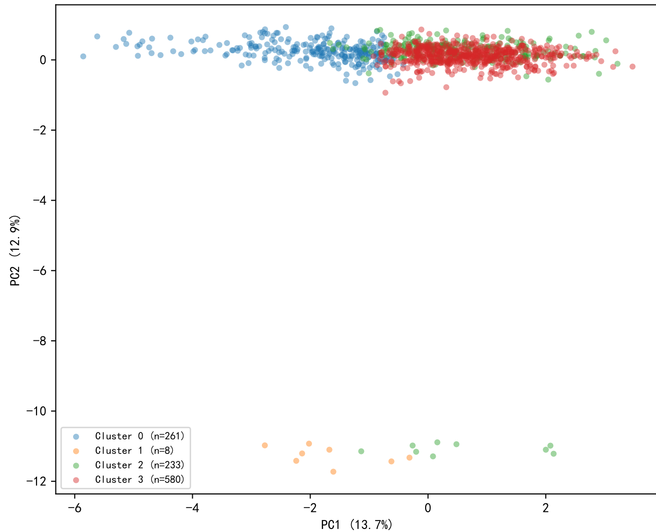
K-Means (k=4) — PCA
