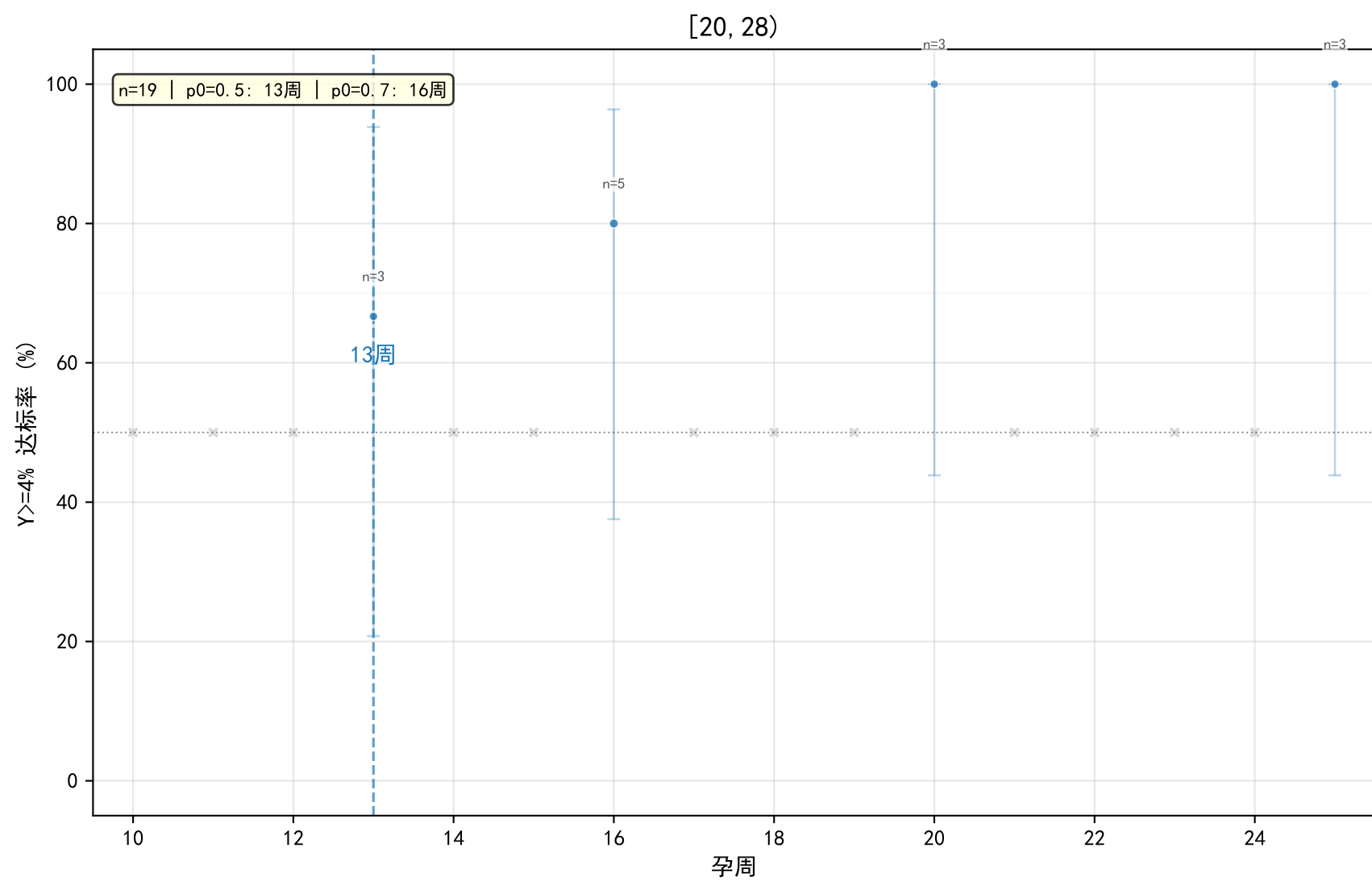
各BMI组达标率 — 直接计数 + Wilson 95%CI + 样本量标注 点大小 \propto \log(n) , n<10 标注数字, 误差棒=95% Wilson CI
