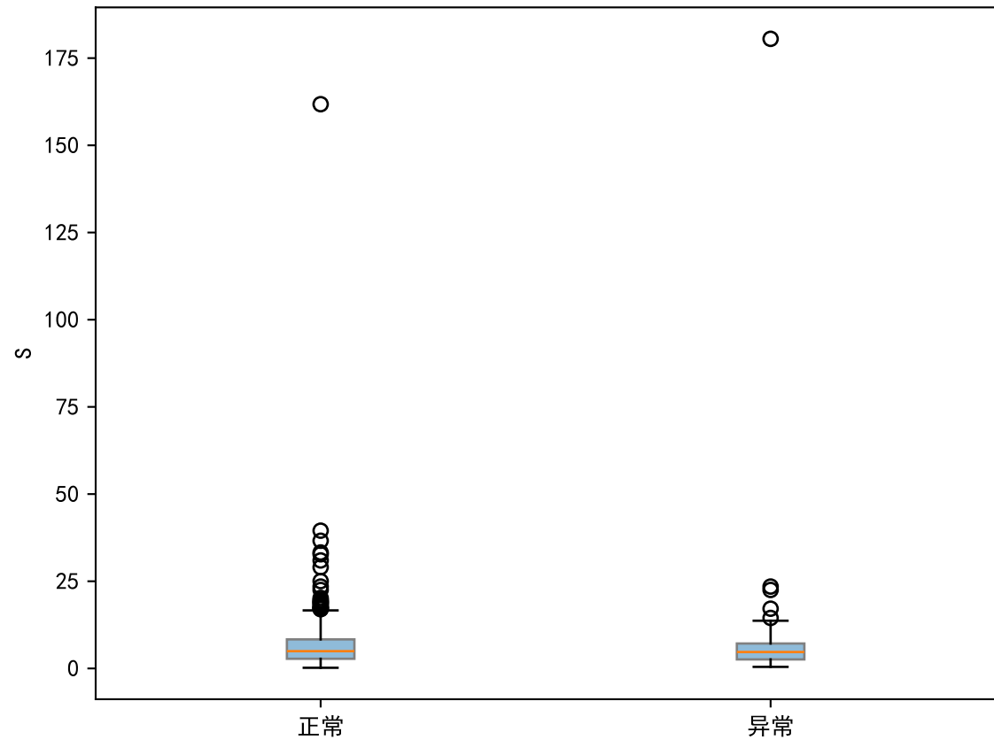
评分箱线图
