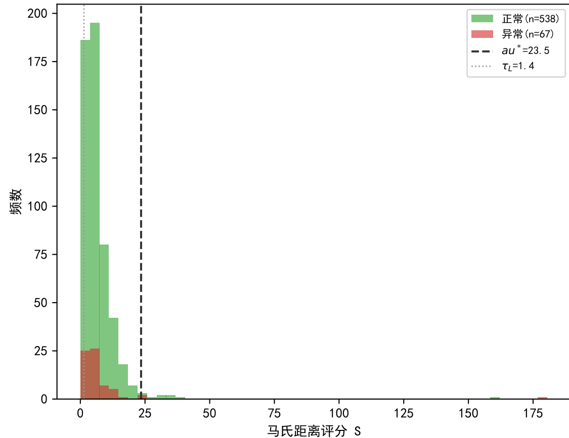
评分分布
