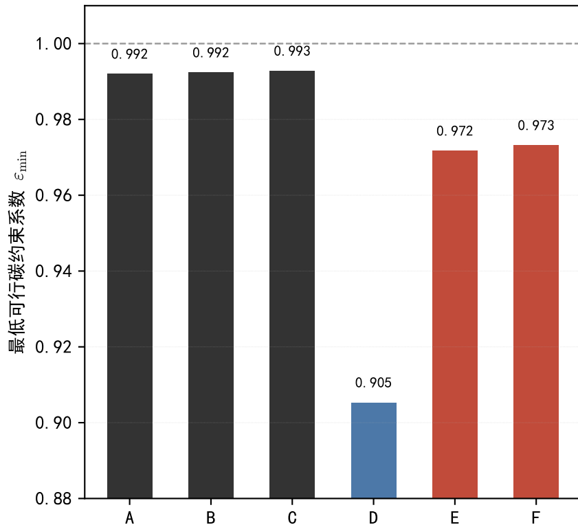
逐区域 \varepsilon_{\min} ：碳约束可行域下限
