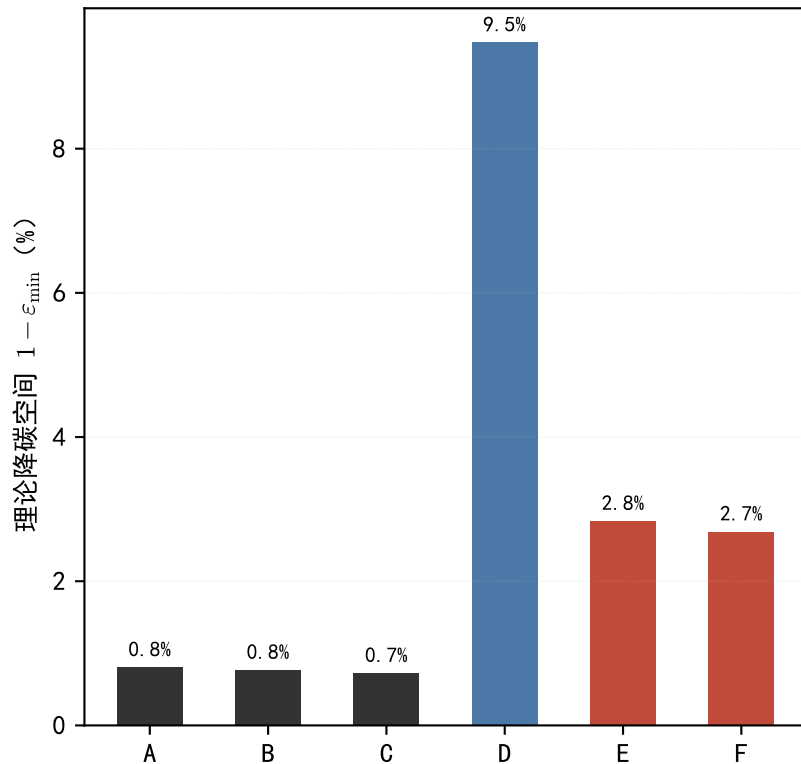
降碳空间：东部 \approx 1\% ，西部绿电 \approx 2.7\% ，D 区 \approx 9.5\%
