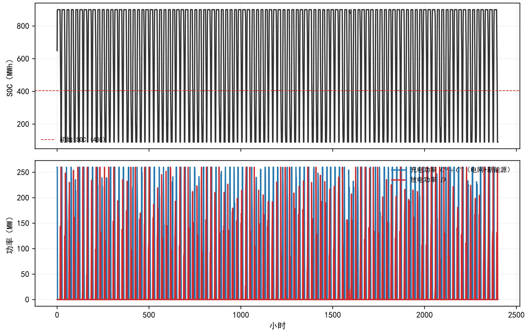
D 区储能荷电状态与充放电（主时域 0-2399h）
