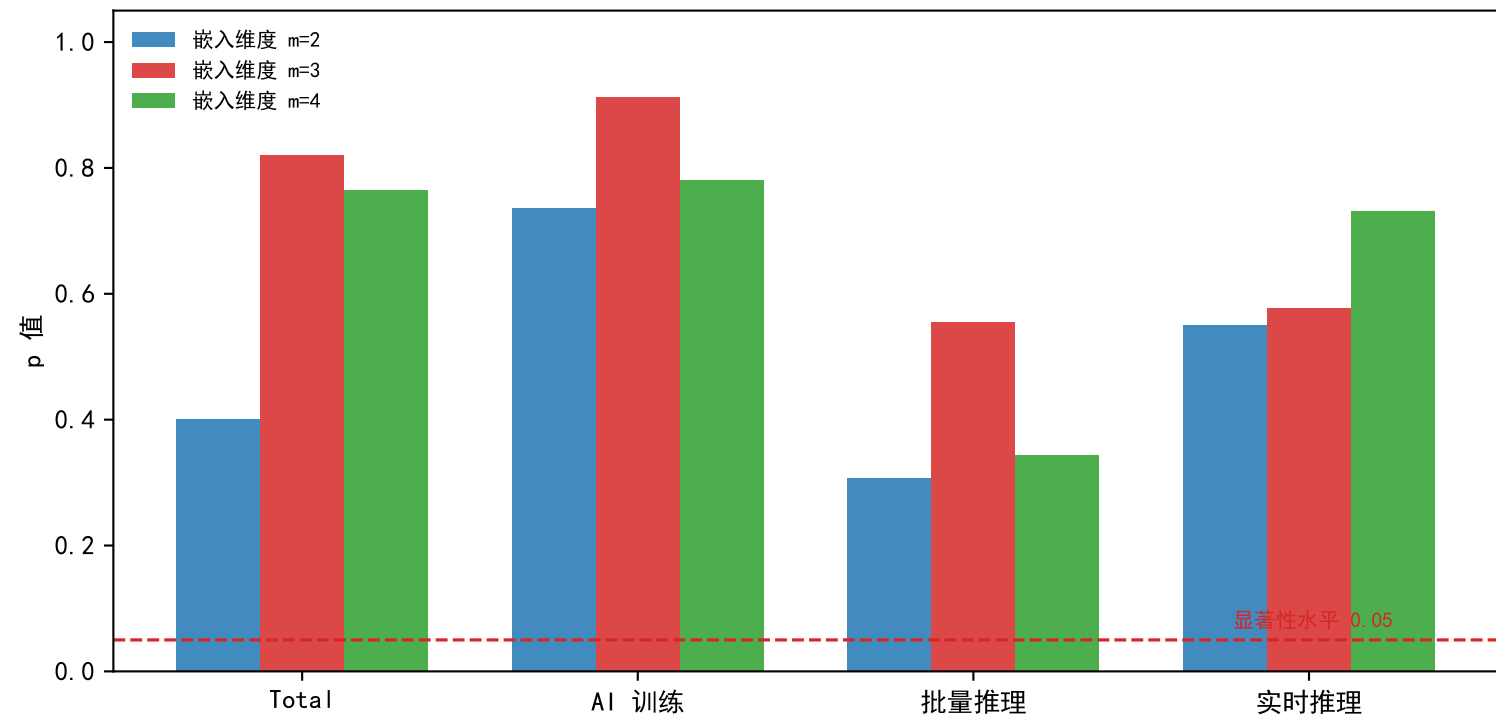
BDS 非线性依赖检验：全部 p \geq 0.30 ，不拒绝 i.i.d.（白噪声）
