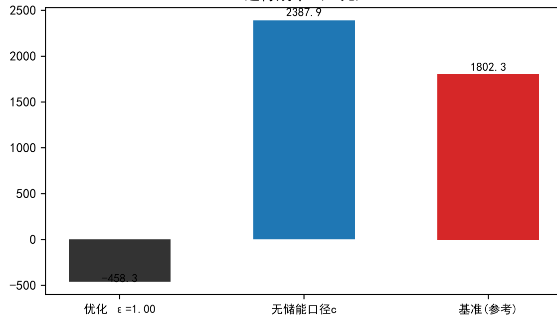
峰值净购电 (MW)
