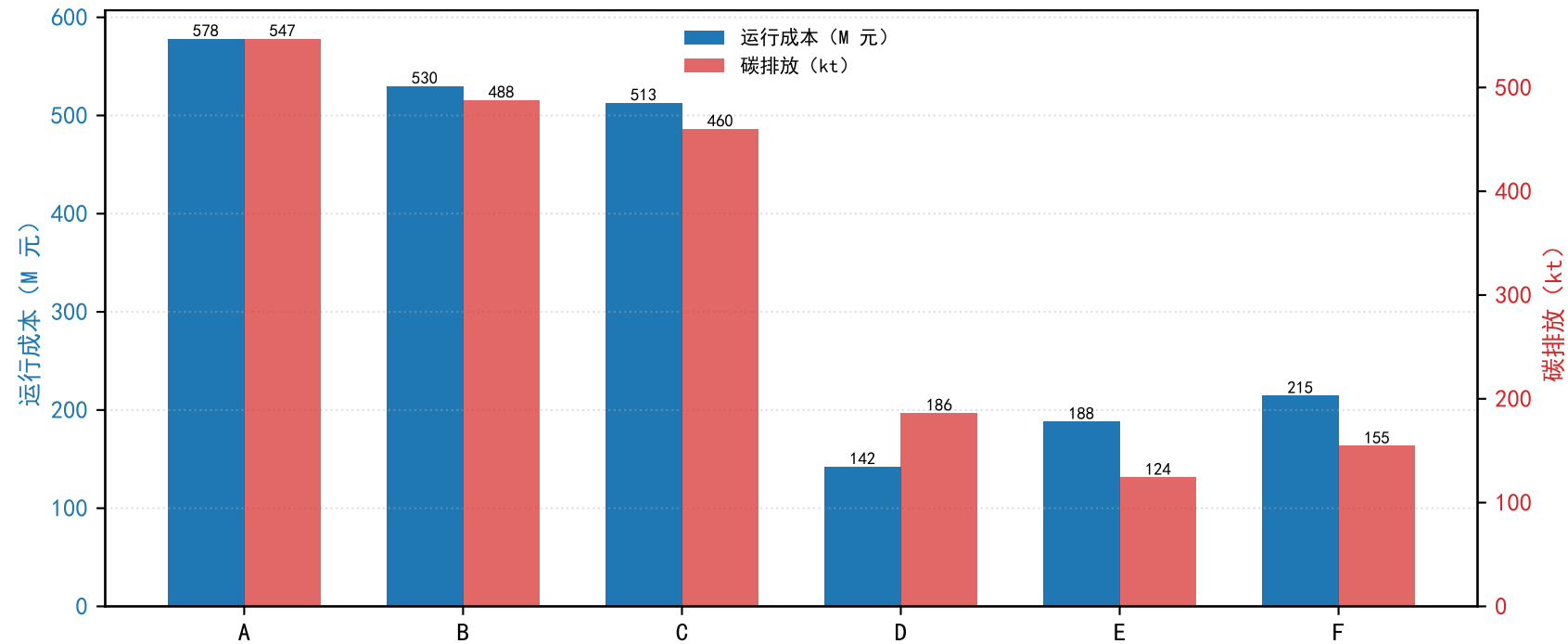
S0 主解：六区域运行成本与碳排放分解（A-F 对应 RegionA-F）
