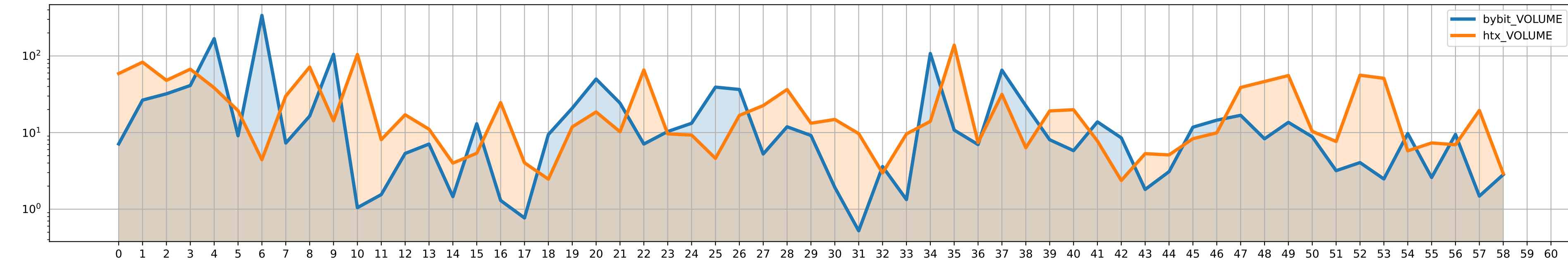
AAVE/USDT volumes
