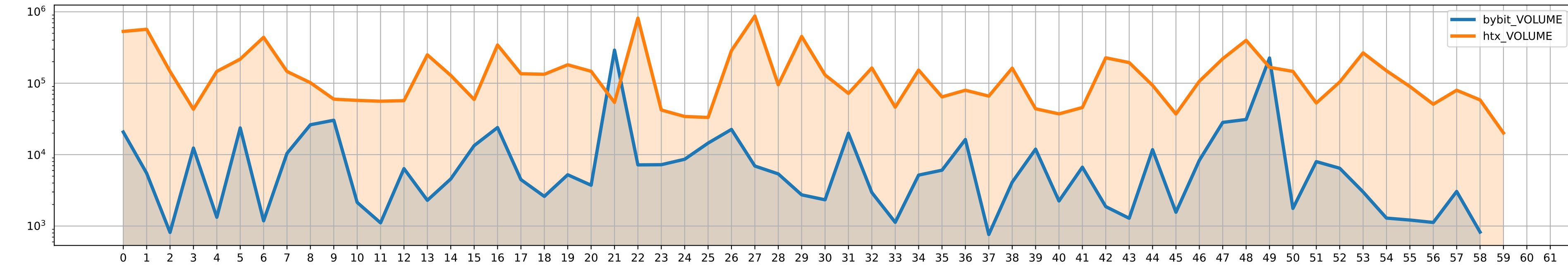
TRX/USDT volumes
