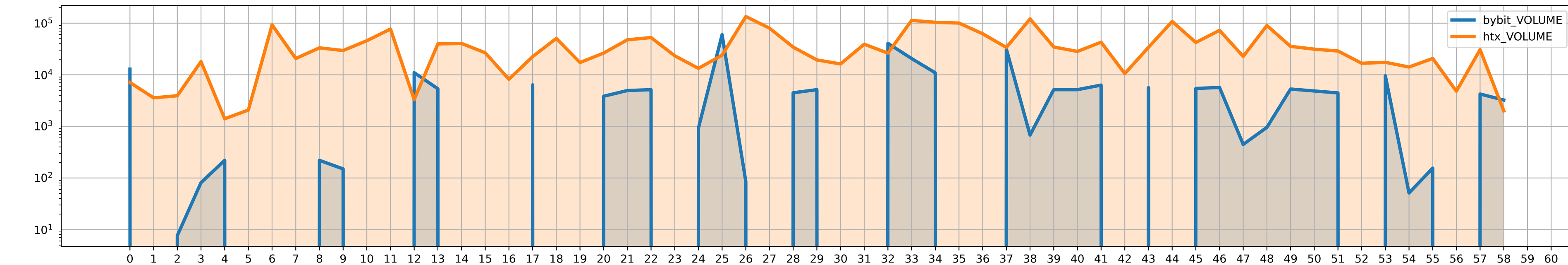
ALGO/USDT volumes
