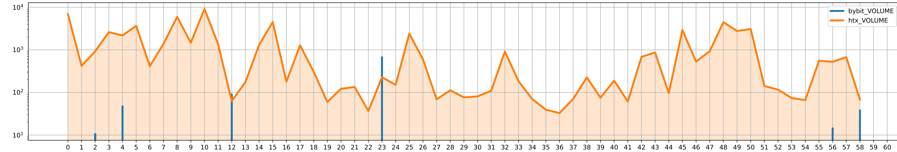
UMA/USDT volumes
