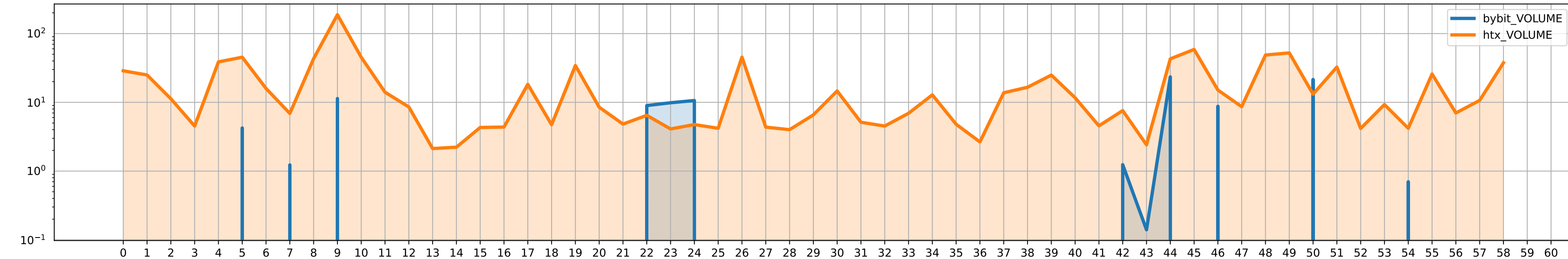
GMX/USDT volumes
