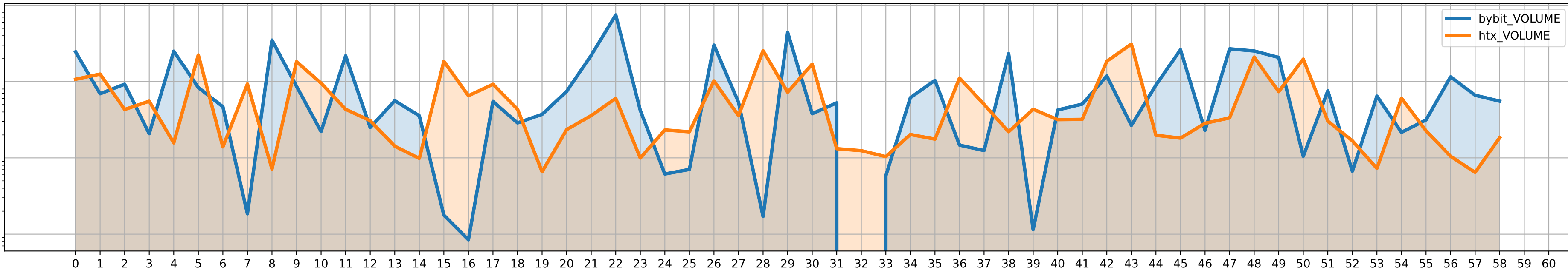
ARB/USDT volumes
