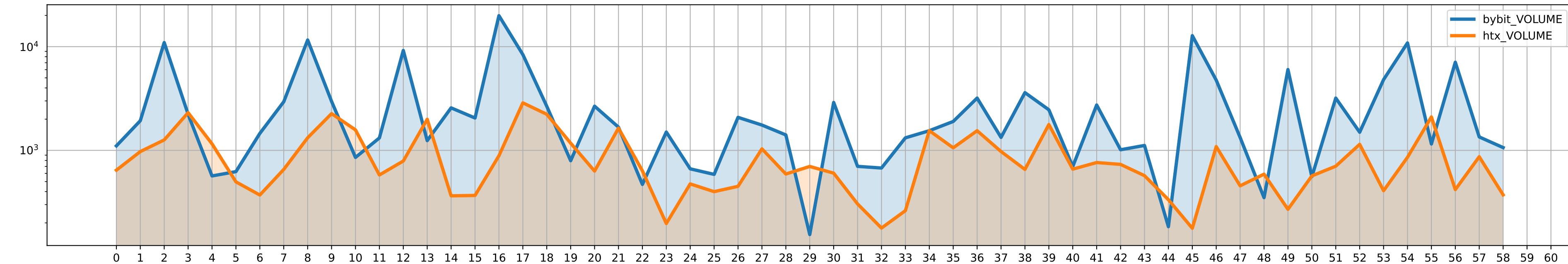
TIA/USDT volumes
