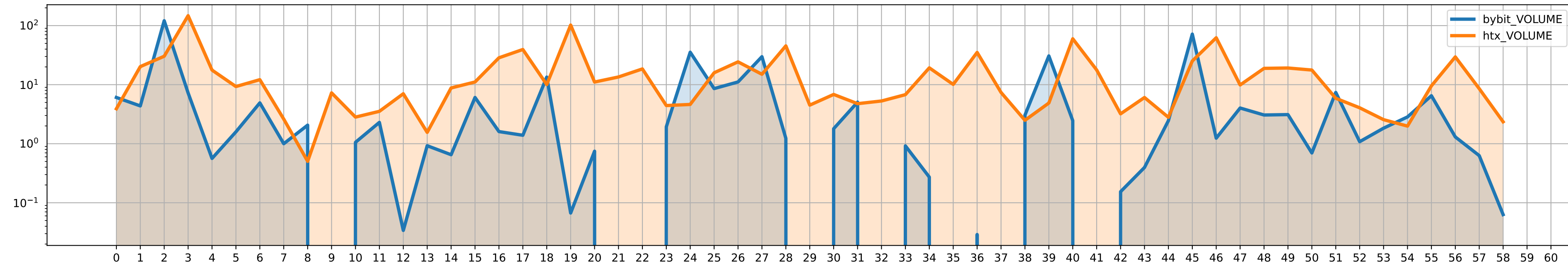
BCH/USDT volumes
