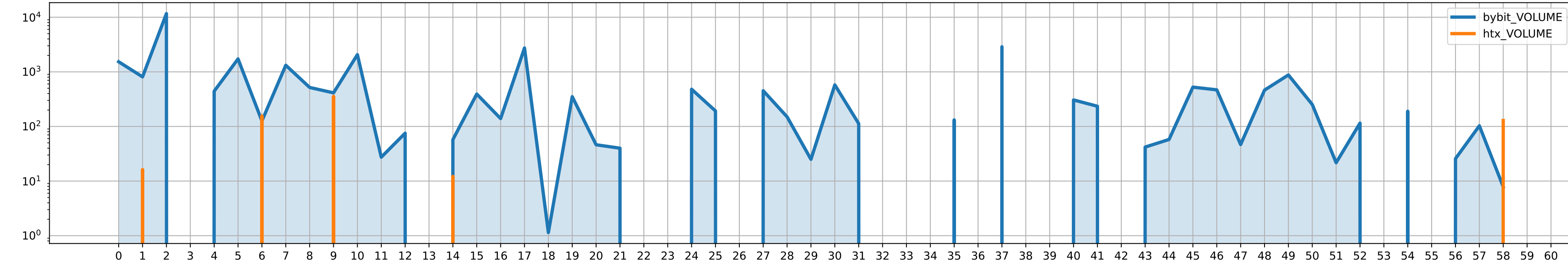
OP/USDT volumes
