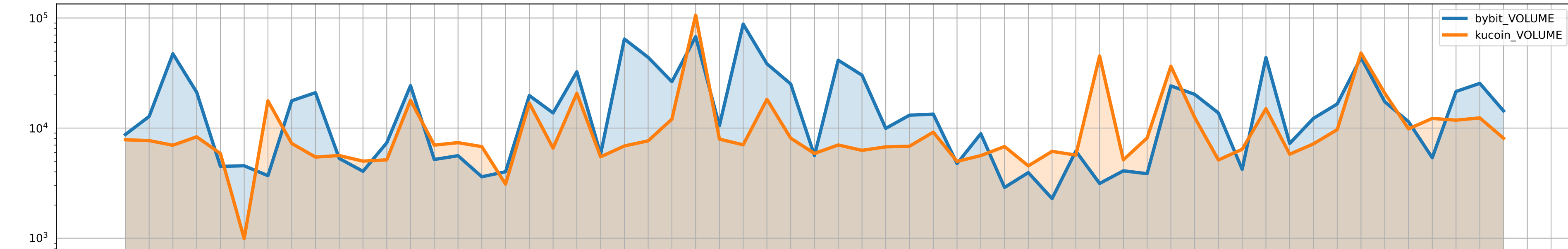
SUI/USDT VOLUMES
