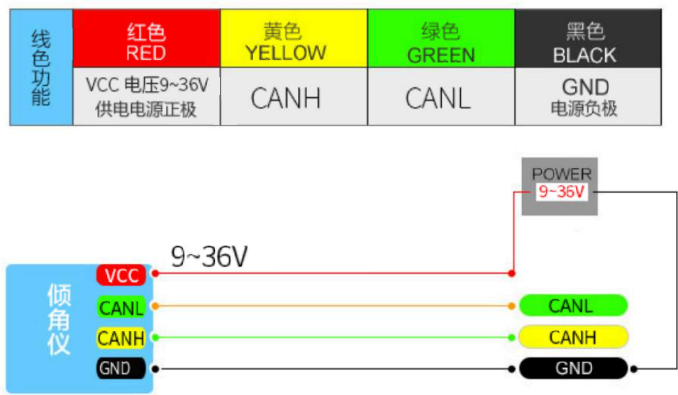
(CAN接线方式)
