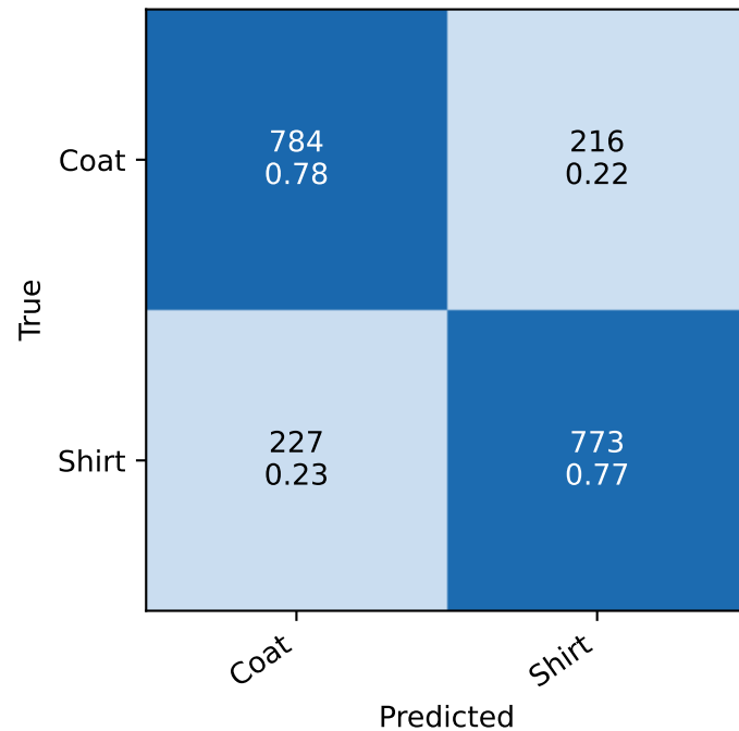
Coarse CNN
