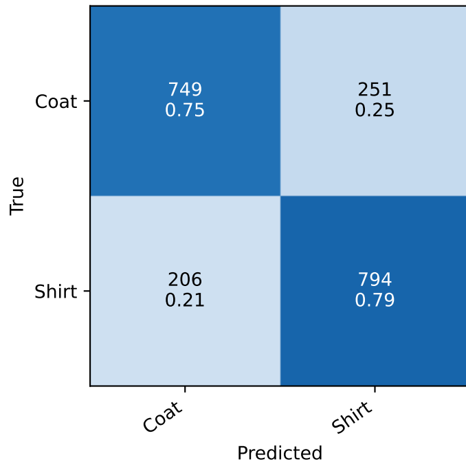
Random CNN
