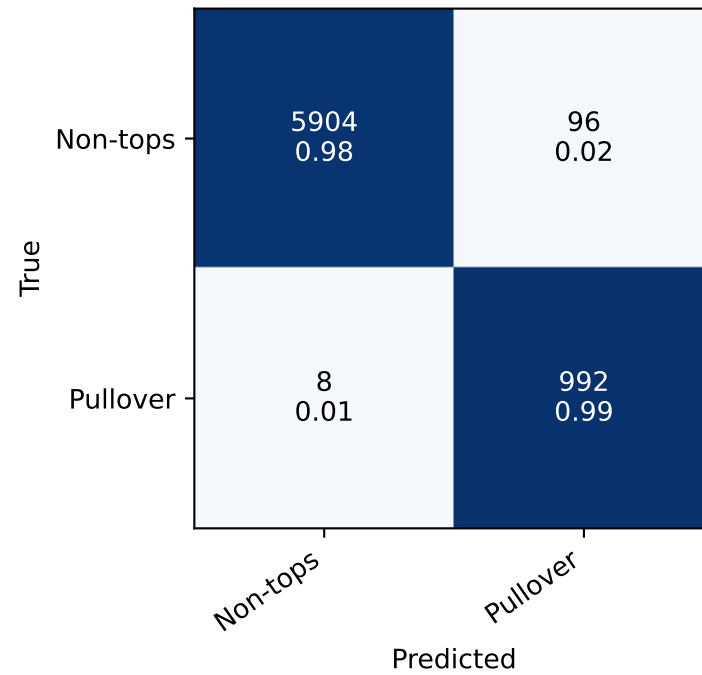
Coarse CNN
