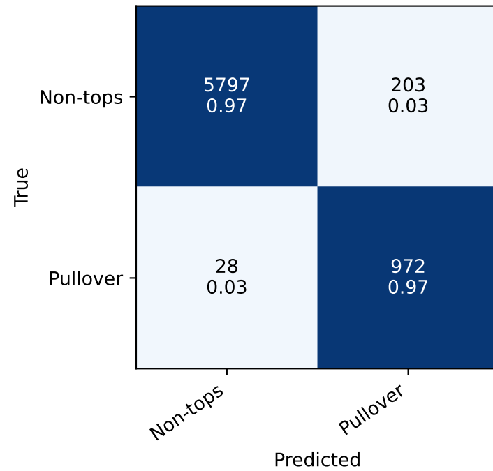
Random CNN
