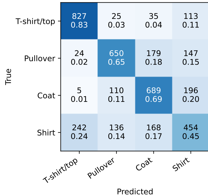
Coarse CNN
