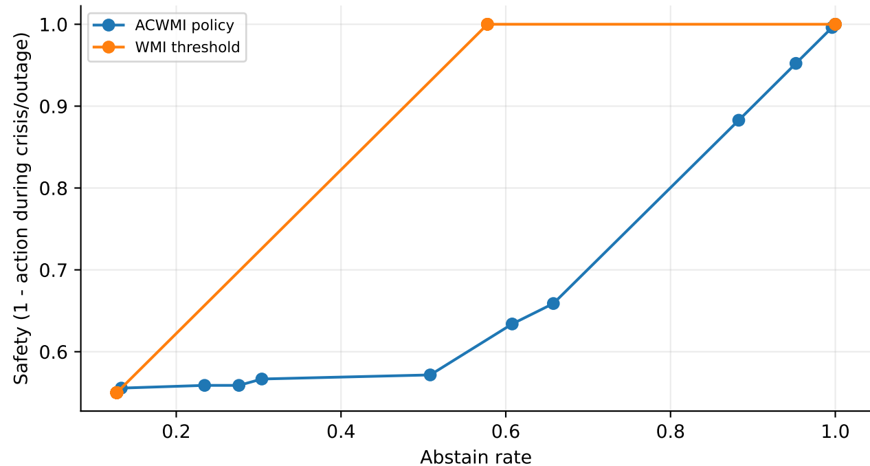
Fig. 7. Pareto frontier: abstention vs stress safety
