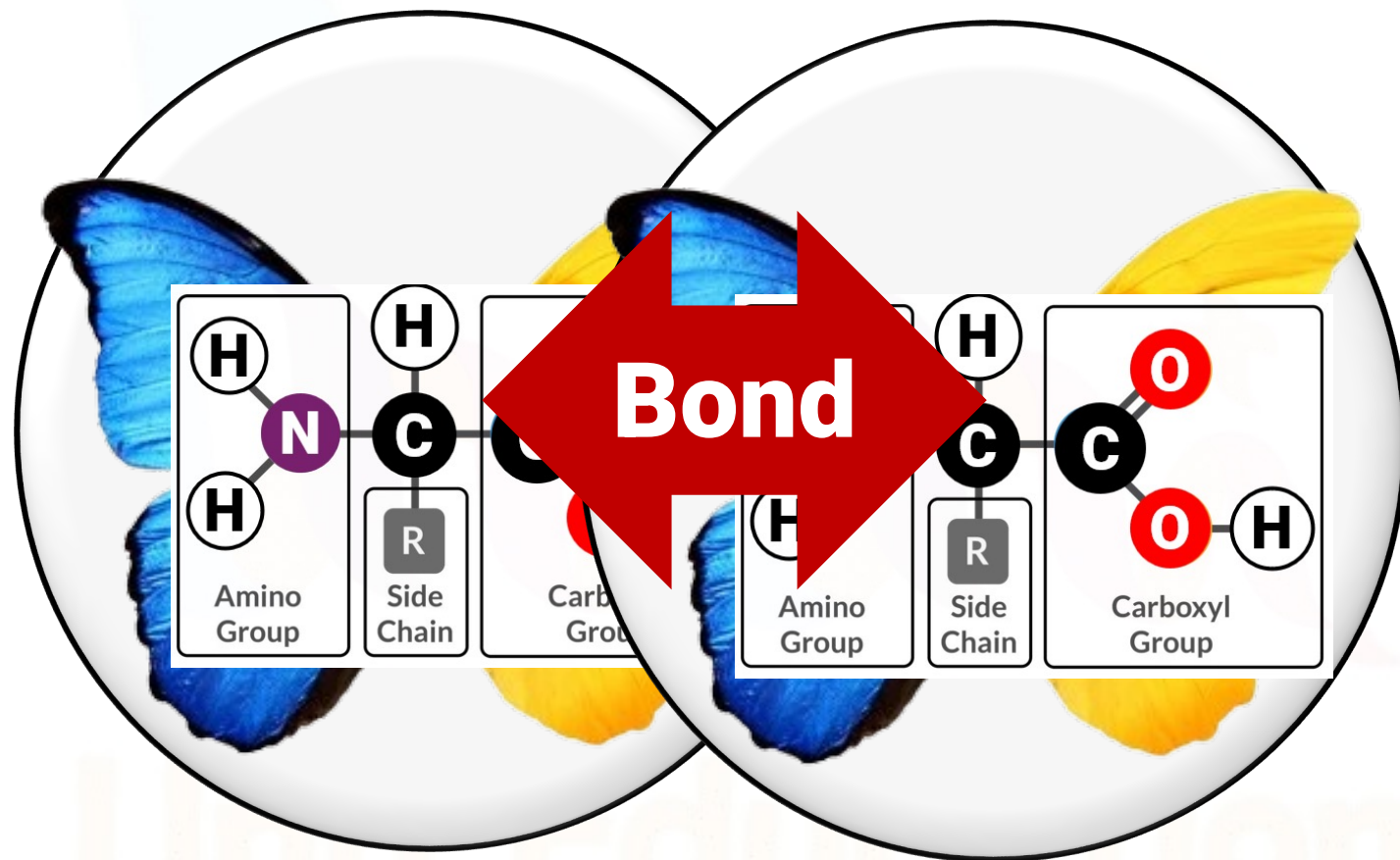
Dipeptide (二肽)
