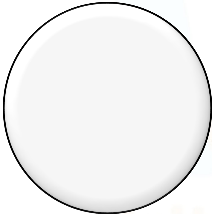
Glycerol (甘油)
