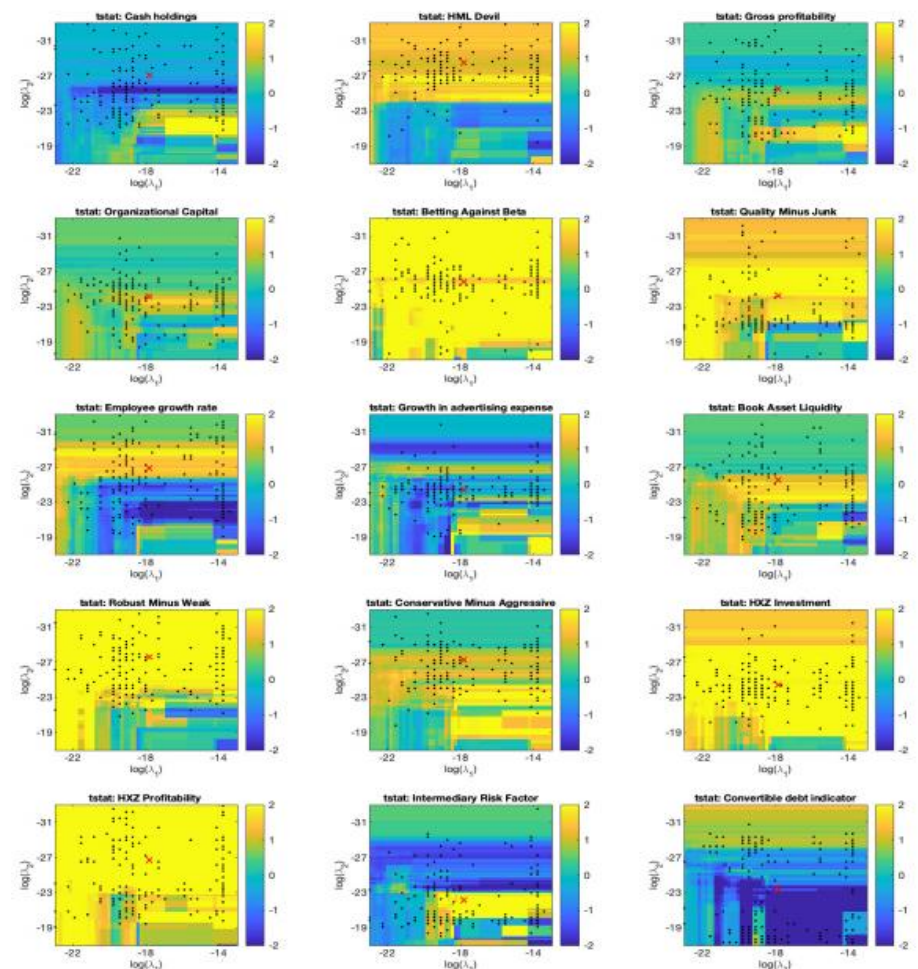
图 4：不同参数下因子显著性热图
