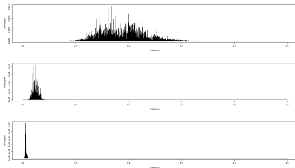
图 6: 高盛指数日度收益率频率强度 (由上到下以此为: 短周期、中周期、长周期)
