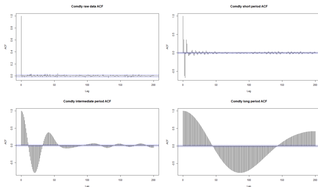
图 3： 高盛商品指数日度收益率自相关性
