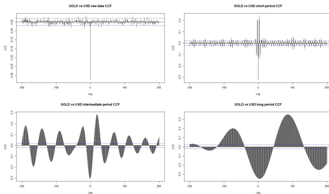
图 9：黄金 vs 美元指数
