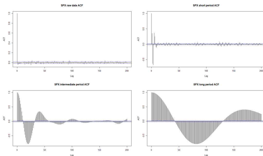
图 2： S&P 500 指数日度收益率自相关性
