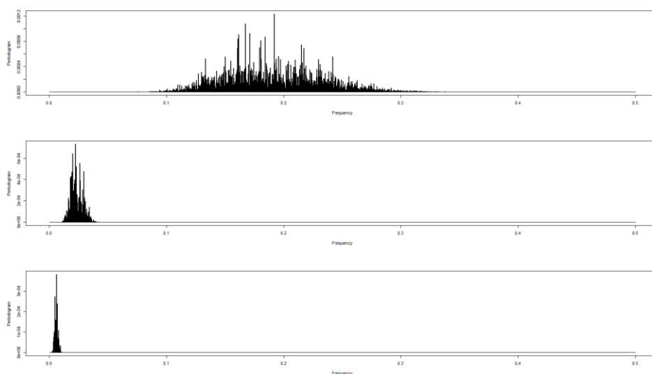
图 4： 黄金日度收益率频率强度（由上到下以此为：短周期、中周期、长周期）
