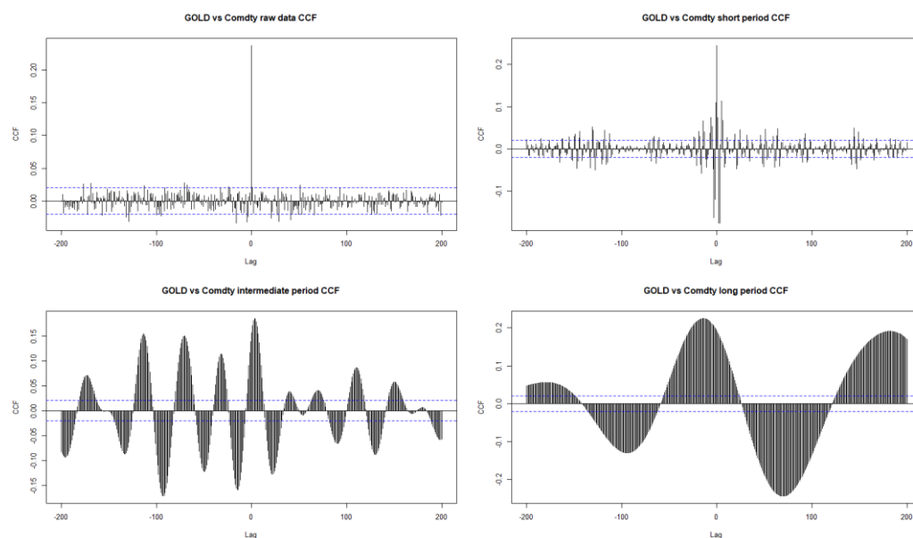
图 8：黄金 vs 高盛商品指数
