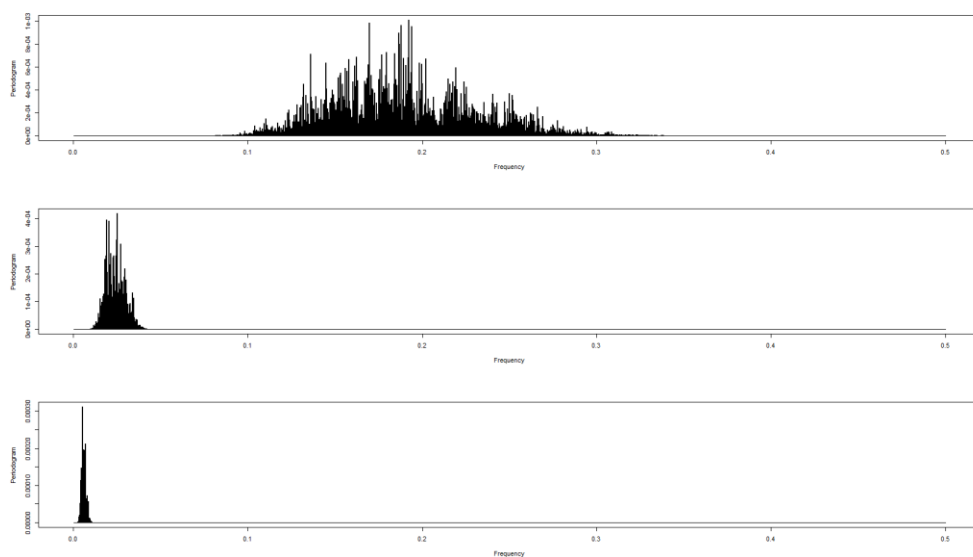
图 5: S&P 500 指数日度收益率频率强度 (由上到下以此为: 短周期、中周期、长周期)
