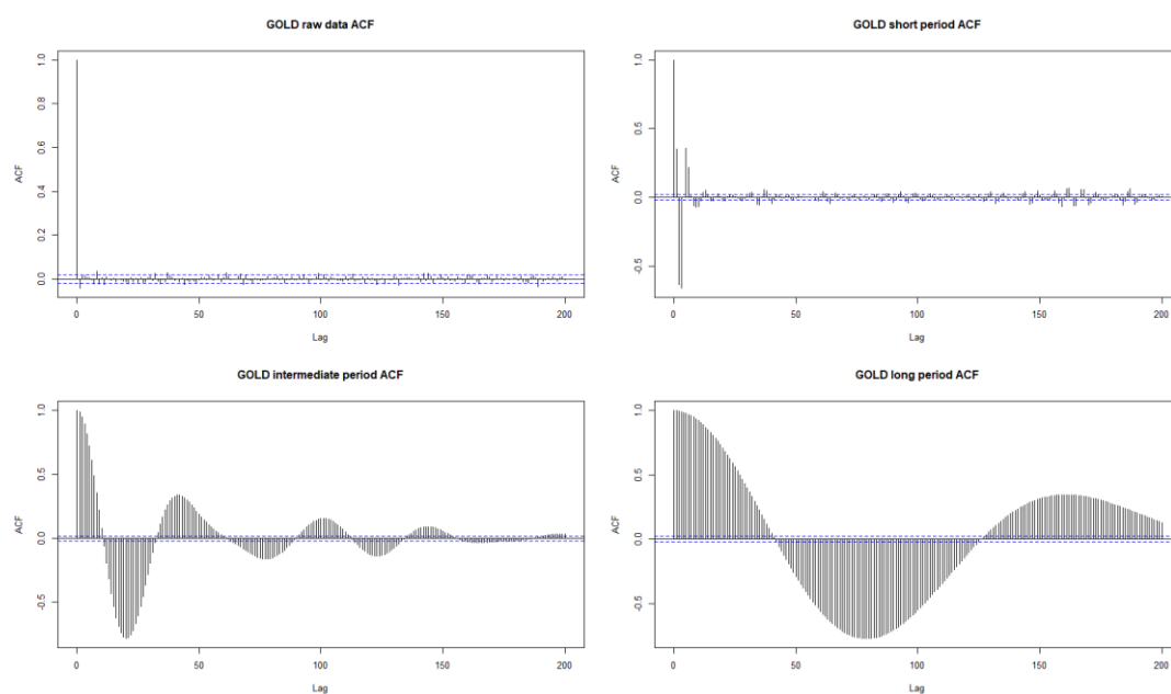
图 1： 金价日度收益率自相关性
