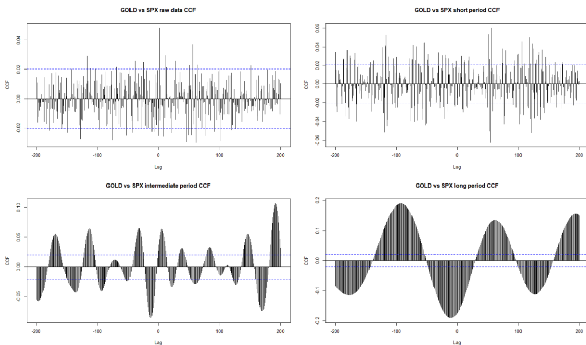
图 7：黄金 vs S&P 500 指数
