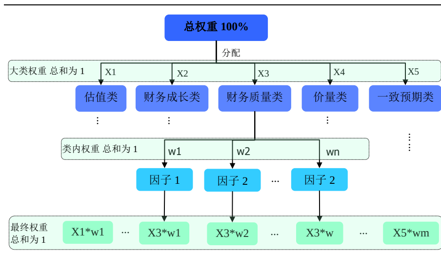
图 1 分层赋权示意图
